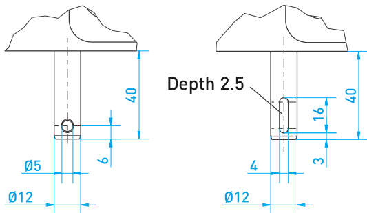
optional crosshole optional keyway
